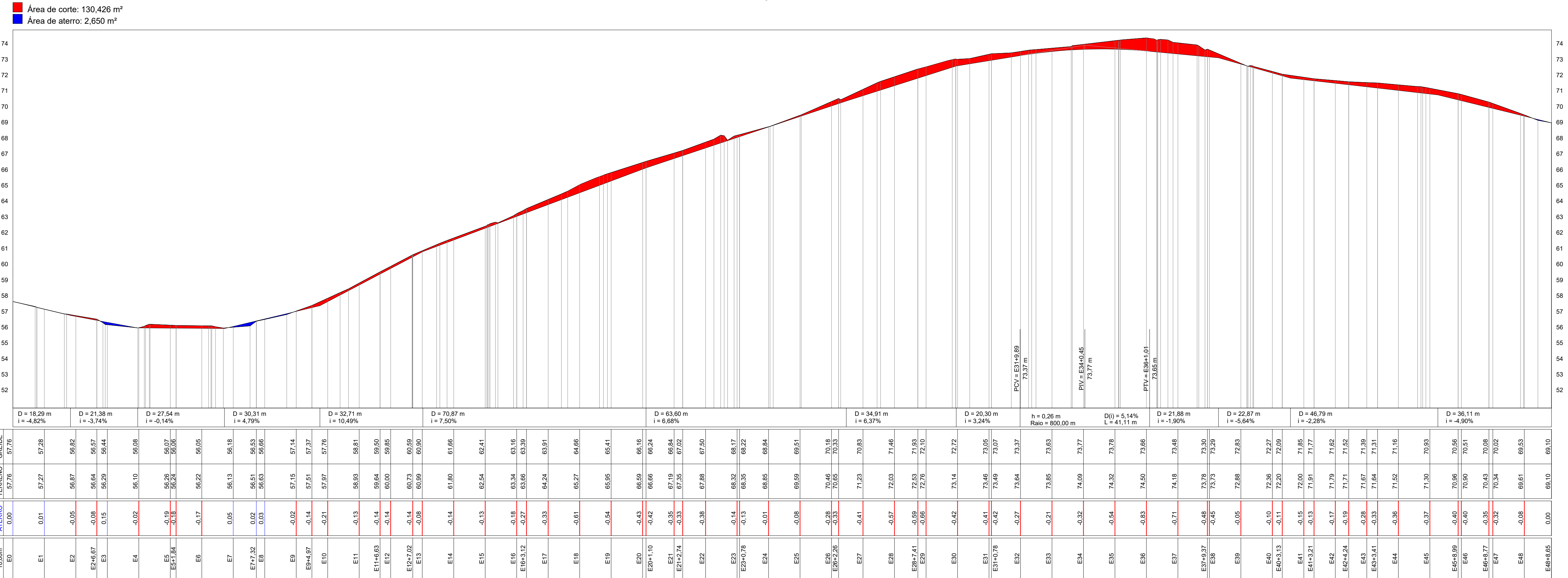
Perfil Longitudinal Trecho 02
